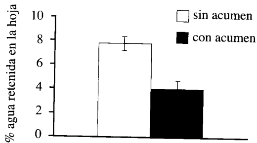
Fig. 1. Porcentaje de agua retenida en la superficie de las hojas antes y después de remover el acumen. Los valores son promedios \pm 1 EE de hojas de 30 especies diferentes (n = 30).
